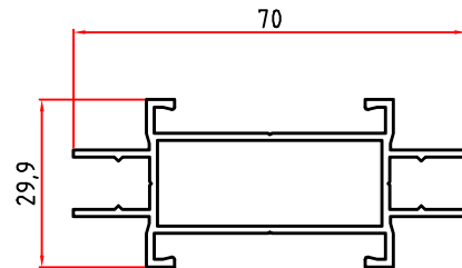
4825 0,811 Kg/m
