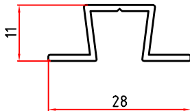
2482 0,170 Kg/m
