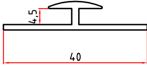
1978 0,248 Kg/m
