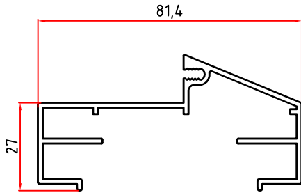
2514 0,974 Kg/m
