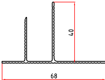
6138 0,435 Kg/m
