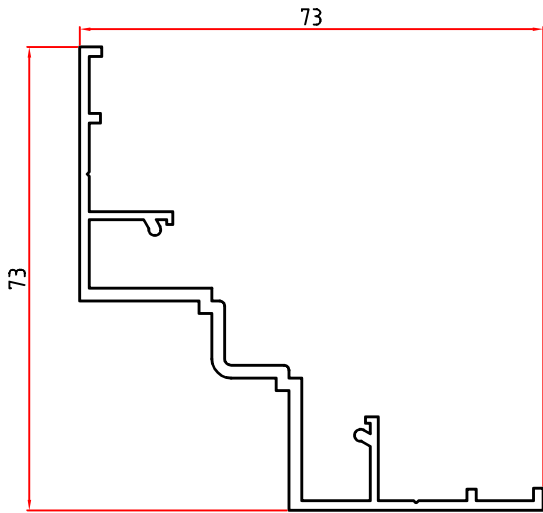
6156 0,861 Kg/m
