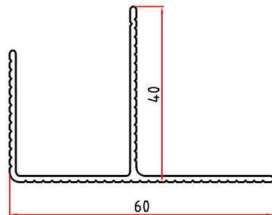
6202 0,479 Kg/m
