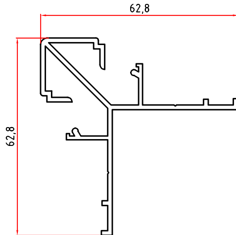
6155 0,857 Kg/m
