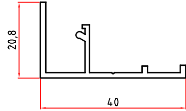
6157 0,331 Kg/m
