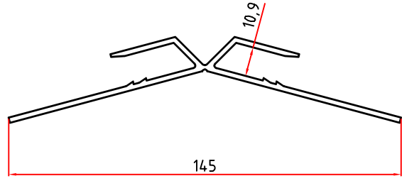
3168 1,279 Kg/m
