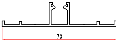
6160 0,453 Kg/m
