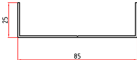
2476 0,489 Kg/m
