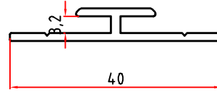
5753 0,248 Kg/m
