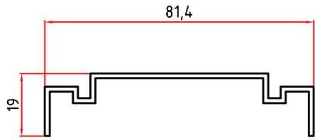
2480 0,556 Kg/m
