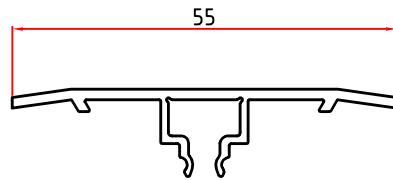
6159 0,336 Kg/m
