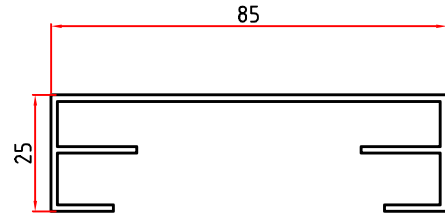
2479 0,757 Kg/m
