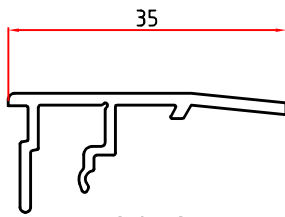
6158 0,255 Kg/m
