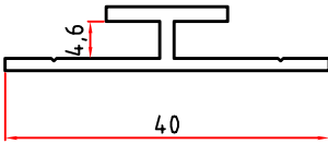
3925 0,271 Kg/m
