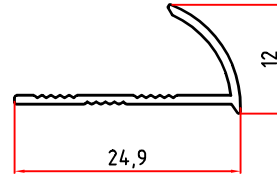
5915 0,098 Kg/m
