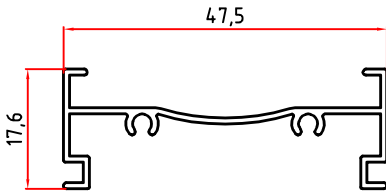
5672 0,288 Kg/m
