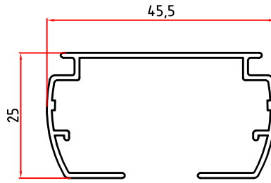
3501 0,371 Kg/m
