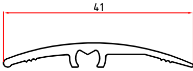
4270 0,230 Kg/m
