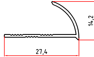
5916 0,114 Kg/m
