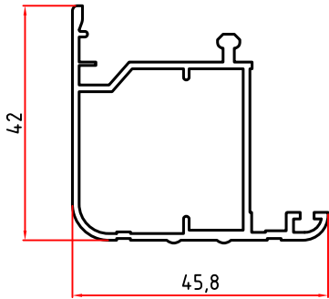
2452 0,627 Kg/m
