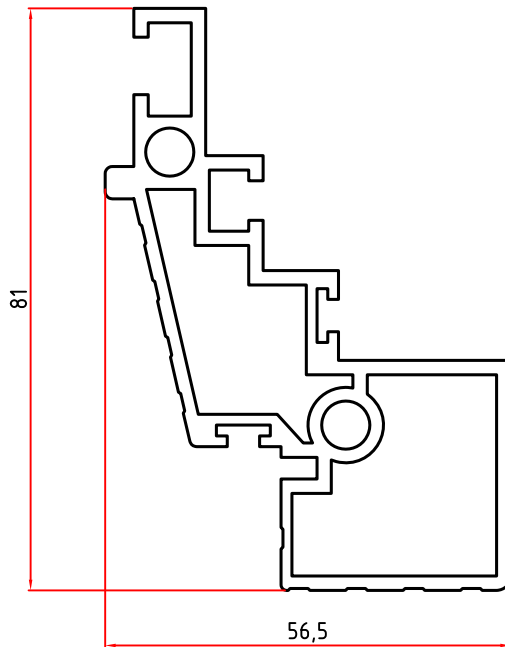
4022 1,808 Kg/m
