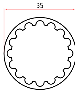
5306 0,690 Kg/m
