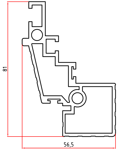
2629 1,829 Kg/m
