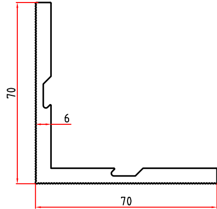
2453 2,053 Kg/m
