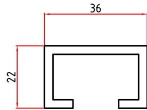
5304 0,751 Kg/m
