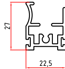
2463 0,502 Kg/m
