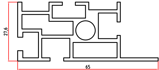
5312 1,180 Kg/m
