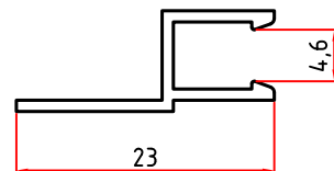
4036 0,118 Kg/m
