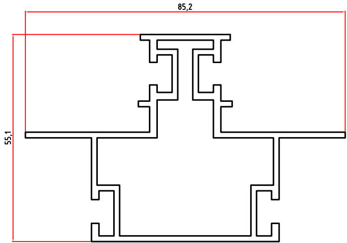
5310 1,385 Kg/m
