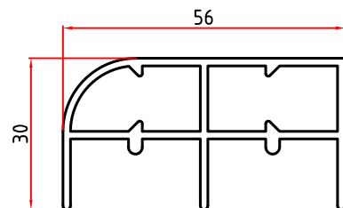
2465 0,878 Kg/m
