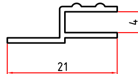
3538 0,110 Kg/m
