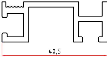
2628 0,563 Kg/m
