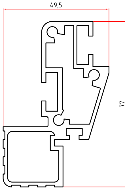
1691 1,849 Kg/m
