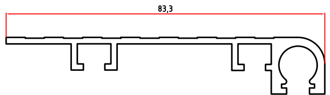
5337 0,721 Kg/m
