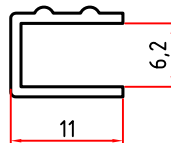
2631 0,084 Kg/m
