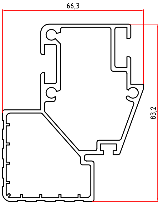
2119 1,932 Kg/m
