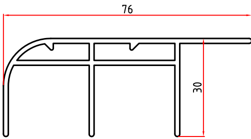
2485 0,882 Kg/m
