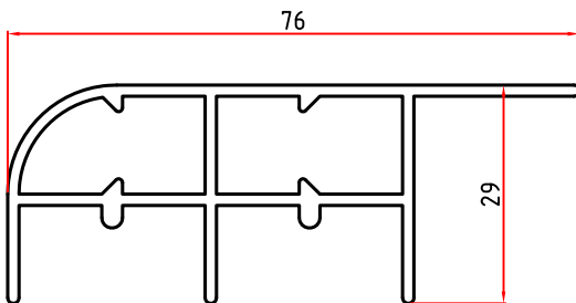
2464 0,941 Kg/m
