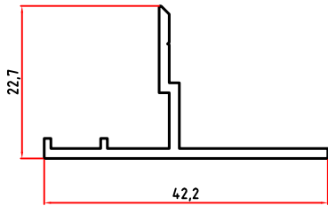
5309 0,283 Kg/m
