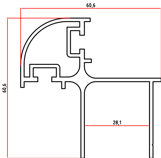
5313 1,118 Kg/m
