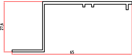
5311 0,353 Kg/m
