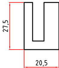
5305 1,175 Kg/m
